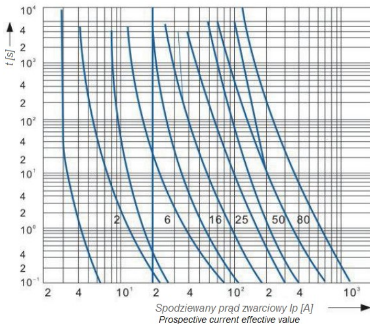
Charakterystyki prądowo-czasowe wkładek topikowych WTS gF Un 500V Time-current characteristics for WTS gF fuse links Un 500V
