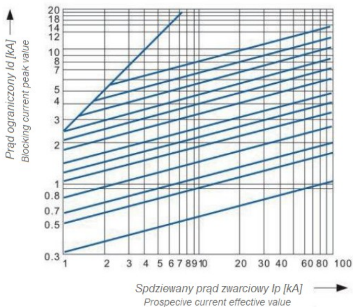
Charakterystyki prądów ograniczonych wkładek topikowych WTS gF Un 500V Blocking current characteristics for WTS fuse links gF Un 500V
